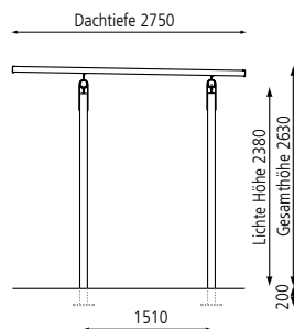
Seitenansicht, einseitig
