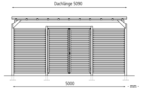
Frontansicht für 4 Stück Abfallgroßbehälter
