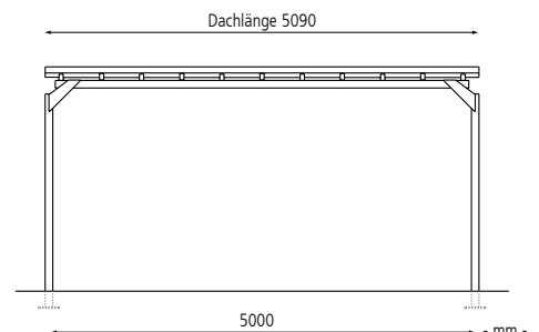
Frontansicht, 1 Feld
